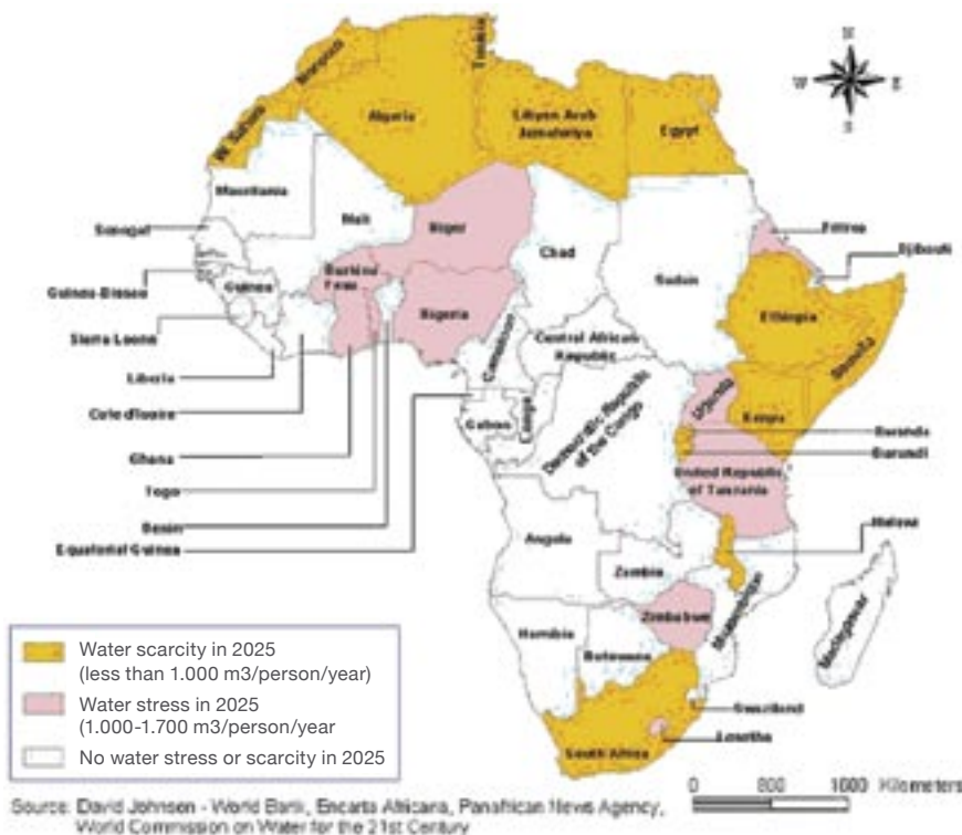
Figur 1. Viser den forventede vandsituation i Afrika. En stor del af Afrika vil opleve alvorlig vandmangel i 2025. Dette skyldes at den globale opvarmning vil intensivere vandets cyklus og forstærke eksisterende mønstre af vandman-
